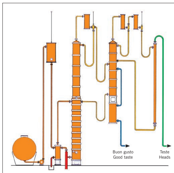
Impianto per brandy / Plant for brandy / Installation pour brandy Instalación para brandy / Anlage für Brandy
