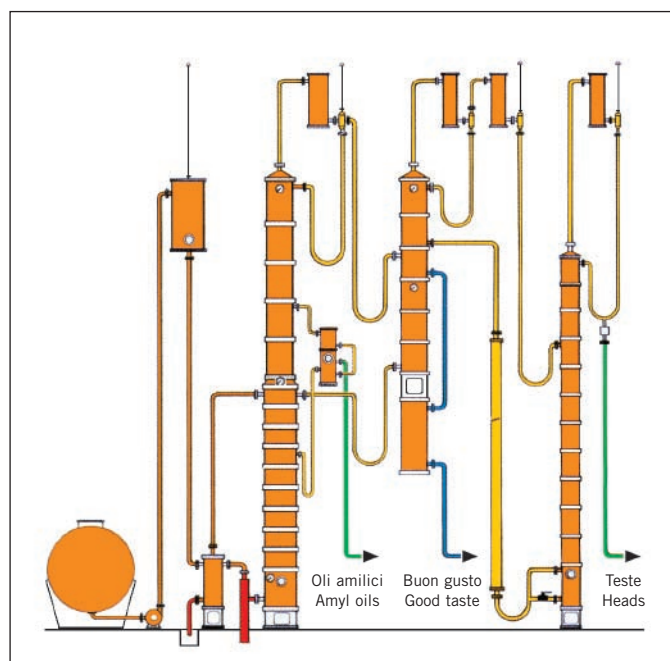
Impianto per grappa / Plant for "grappa" / Installation pour schnaps Instalación para aguardiente / Anlage für Grappa
